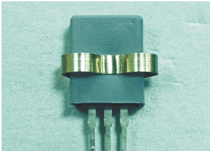
TO220-2 结构图
